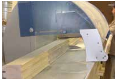
CNC-gesteuerte Blockbohlenbearbeitung
